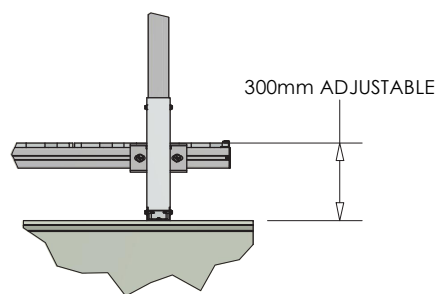
DETAIL Z ( 1 : 20 )
