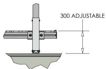
DETAIL Z ( 1 : 20 )
