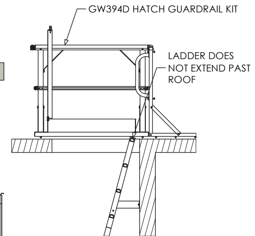
SECTION A-A ( 1 : 40 )
