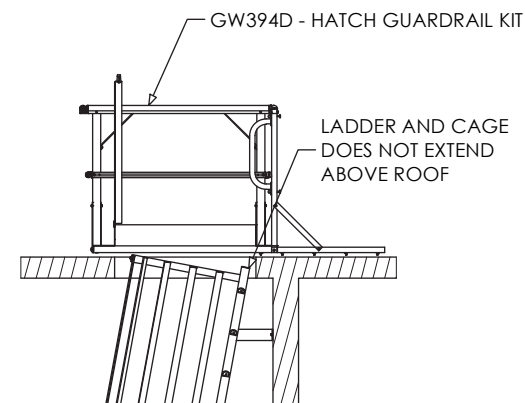
SECTION A-A ( 1 : 50 )
