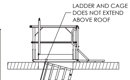
SECTION A-A ( 1 : 60 )
