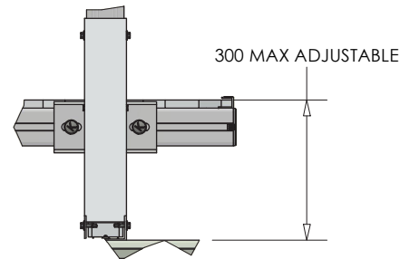
DETAIL Z ( 1 : 10 )
