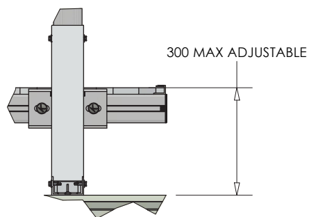
DETAIL Z ( 1 : 10 )
