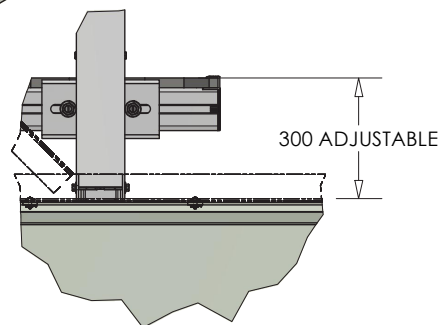
DETAIL Z ( 1 : 10 )
