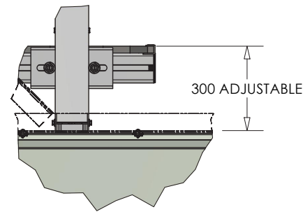
DETAIL Z ( 1 : 10 )
