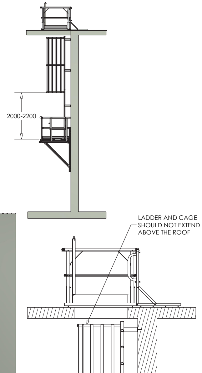
SECTION A-A ( 1 : 40 )
