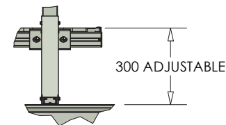
DETAIL Z ( 1 : 20 )
