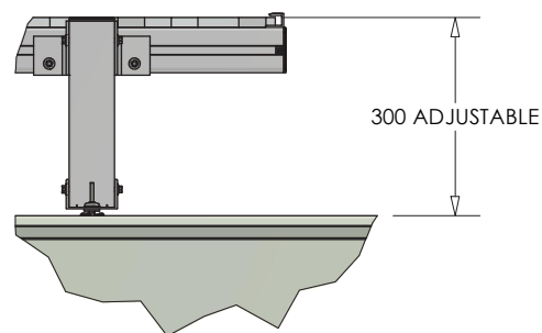
DETAIL Z ( 1 : 10 )
