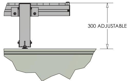
DETAIL Z ( 1 : 10 )
