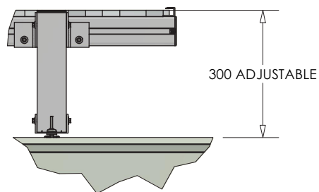
DETAIL Z ( 1 : 10 )
