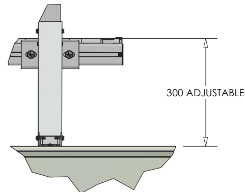
DETAIL Z ( 1 : 10 )
