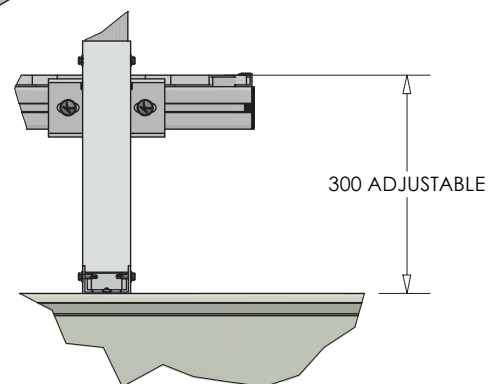
DETAIL Z ( 1 : 10 )
