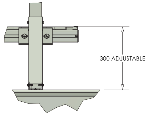
DETAIL Z ( 1 : 10 )
