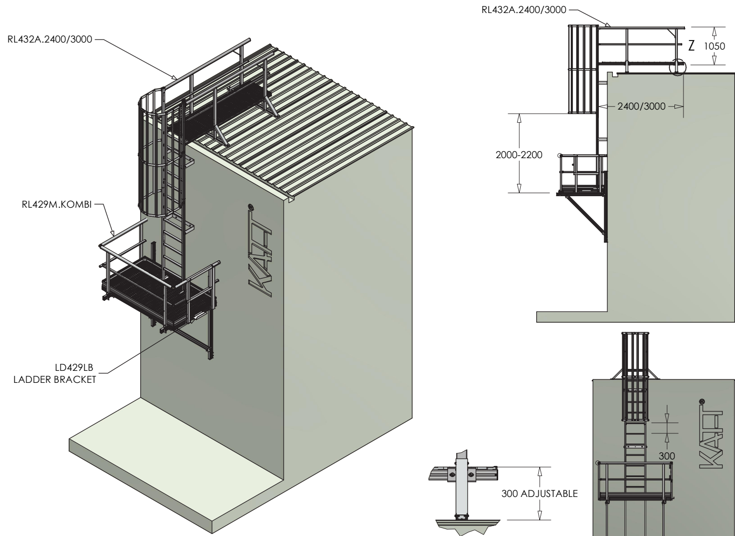
DETAIL Z ( 1 : 20 )
