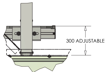
DETAIL Z ( 1 : 10 )
